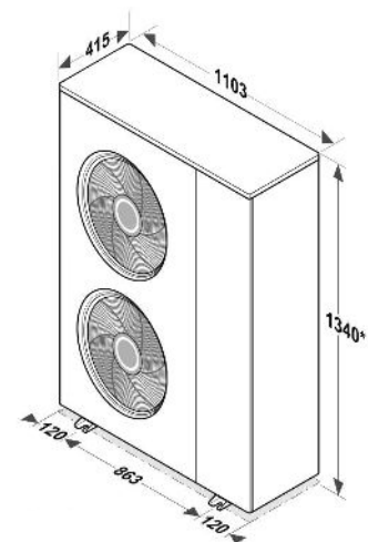
Genia Air 15 Unidad exterior
